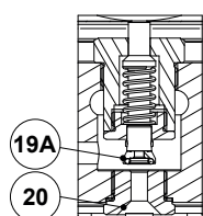
Détail A Vanne pilote (souple)
