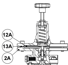
Membrane basse pression en option
