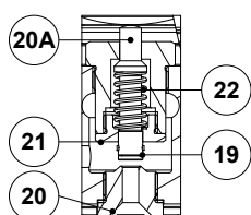
Détail A Vanne pilote
