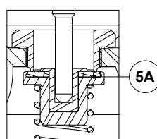
Détail B Vanne principale (souple)
