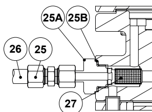
Raccord de prise de pression externe en option
