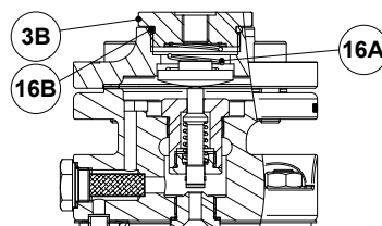
Chargement par dôme en option
