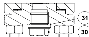
Détail C Raccord de vidange optionnel
