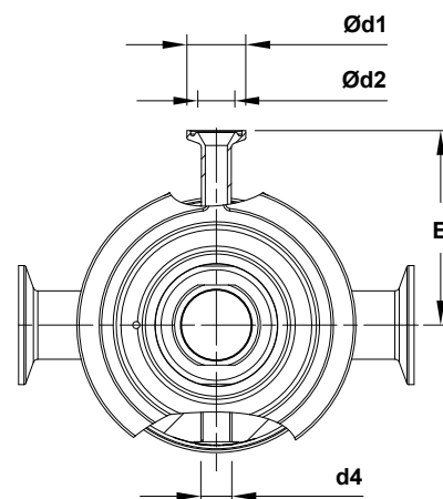
Conexión opcional para manómetro
