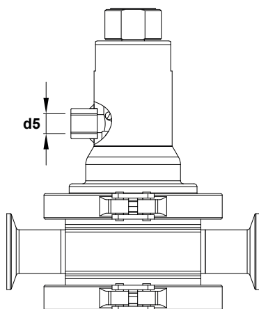
Conexión opcional para línea de fuga
