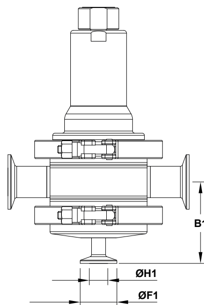
Couvercle inférieur en option avec raccordement de vidange
