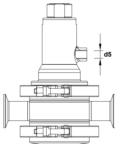
Raccordement optionnel de la ligne de fuite
