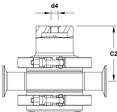
Chargement par dôme en option
