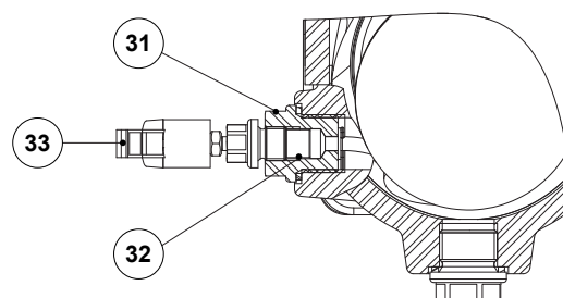
Palanca de elevación del flotador opcional (FLL)
