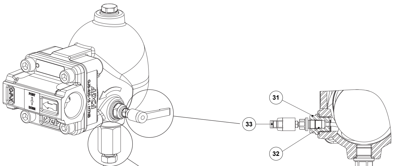
Levier de levage du flotteur optionnelle (FLL)
