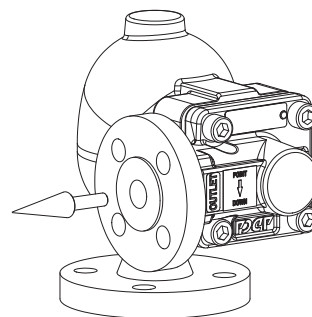
VL - Entrada vertical / salida lateral izquierda
