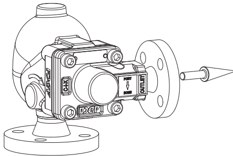
VR - Entrada vertical / salida lateral derecha
