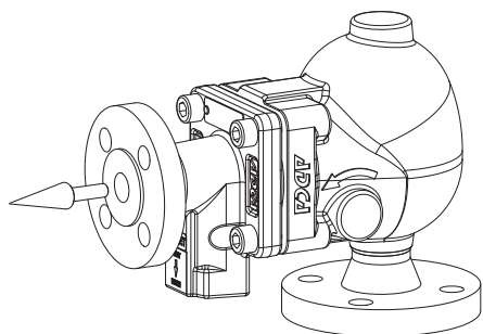
VF - Entrada vertical / salida frontal en línea recta
