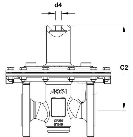
Optional dome-loading
