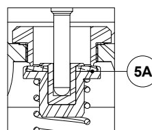
Détail B Vanne principale (souple)
