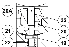
Détail A Vanne pilote
