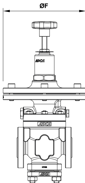
Optional low pressure top
