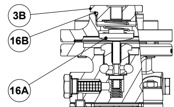
Optional dome-loading
