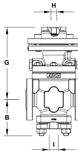
Optional dome-loading
