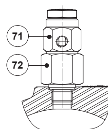
VB21M - Автоматический прерыватель вакуума
