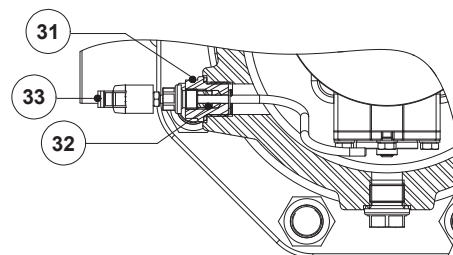
FLL - Устройство для принудительного открытия
