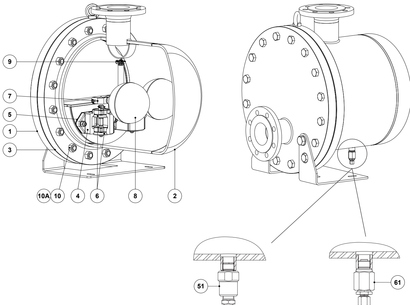
Vanne de purge optionnelle (BDV); Manuelle
