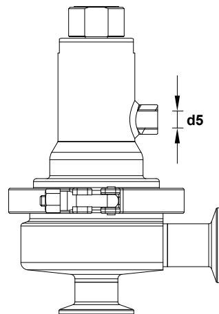
Conexión opcional para línea de fugas
