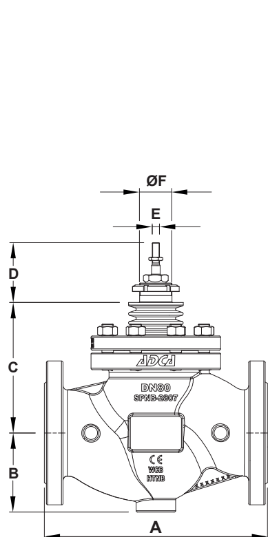
Vanne avec chapeau standard
