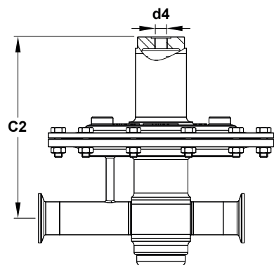
Optional dome-loading
