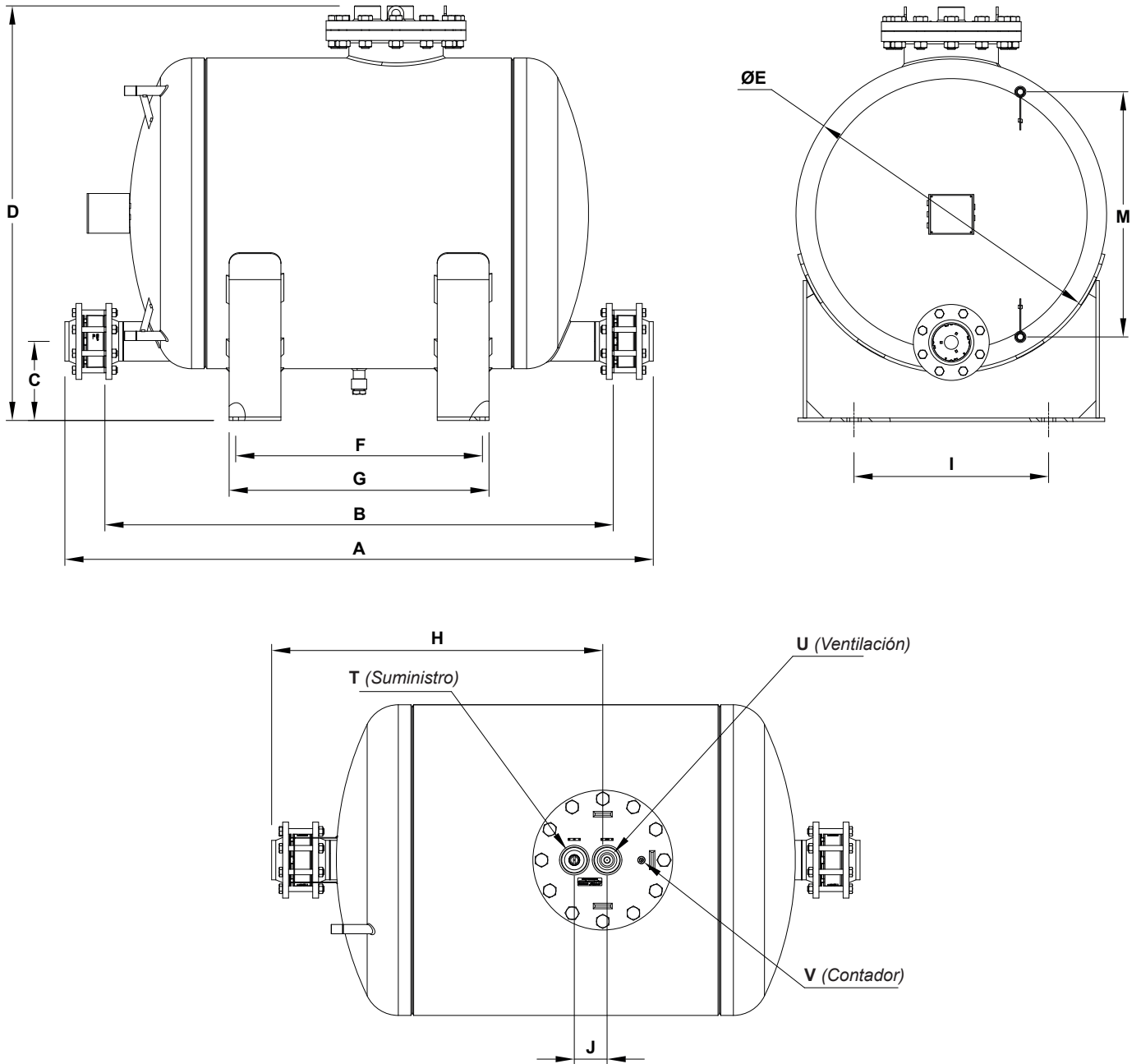
DIMENSIONES (mm)
