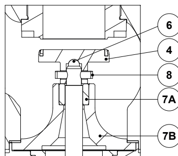
Détail A (2" et 21/2")
