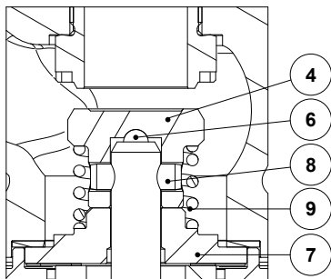
Détail A (1/2" à 11/2")
