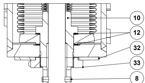
Détail C (6")
