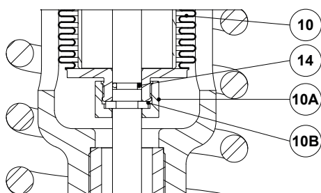
Détail B (3" et 4")
