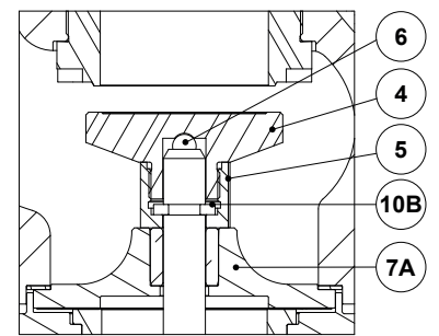
Détail A (3" et 4")
