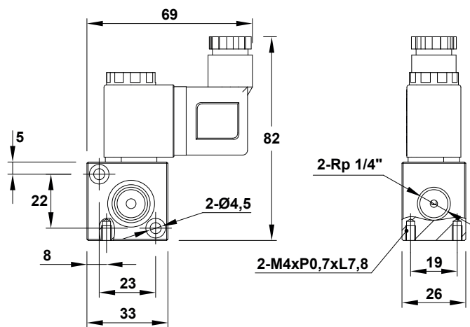
SV32C
