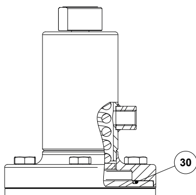
Raccordement de la ligne de fuite (en option)
