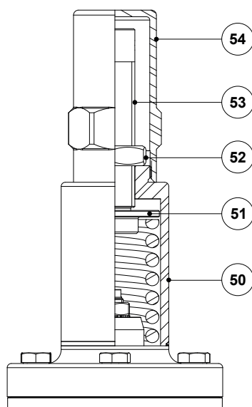
Bouchon supérieur (Optionnel)
