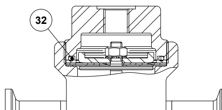
Carga por domo opcional
