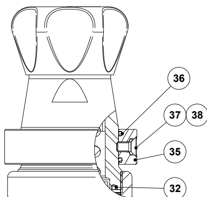
Conexión de la línea de fuga opcional
