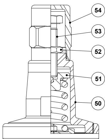
Tapa superior opcional
