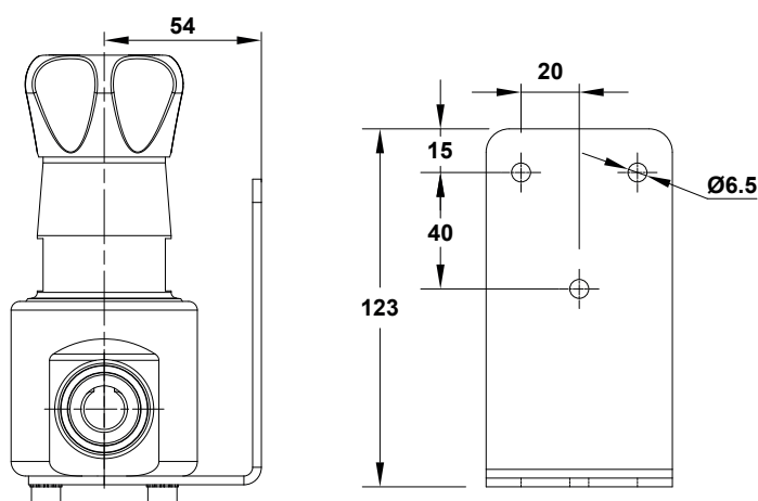
Montaje en la pared opcional
