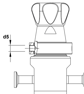
Conexión de la línea de fuga opcional
