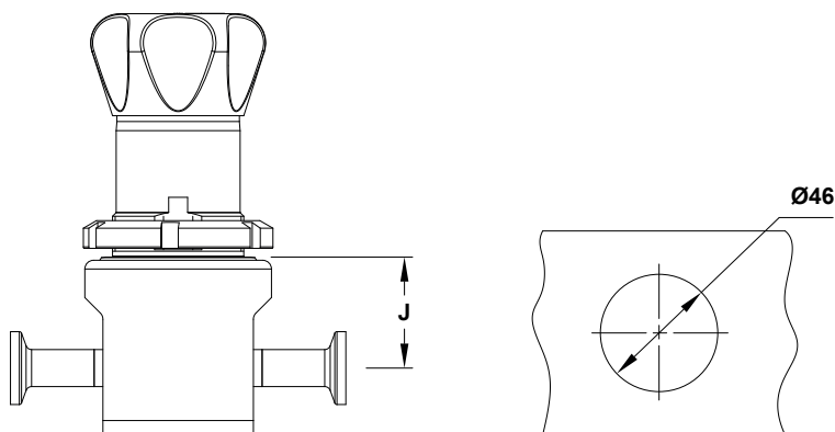
Montaje en panel opcional
