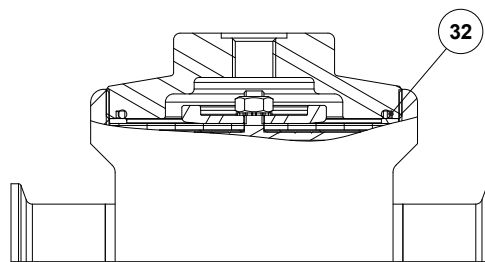
Chargement en dôme optionnel
