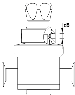
Raccordement de la ligne de fuite (en option)
