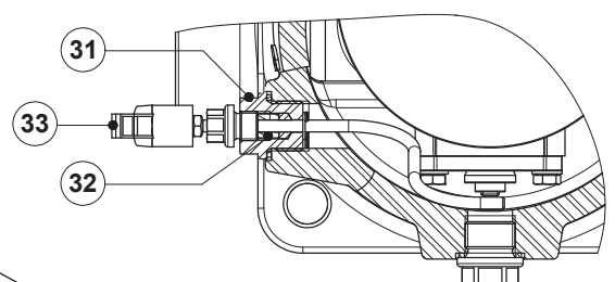
FLL - Anlüfthebel Kugelschwimmer
