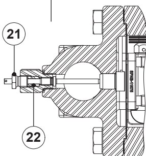
SLR - Bypass-Ventil gegen Dampfabschluss
