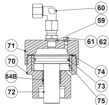
Antrieb P-serie
