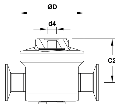
Optional dome-loading
