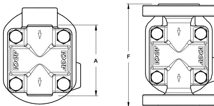
Instalación Vertical (V)
